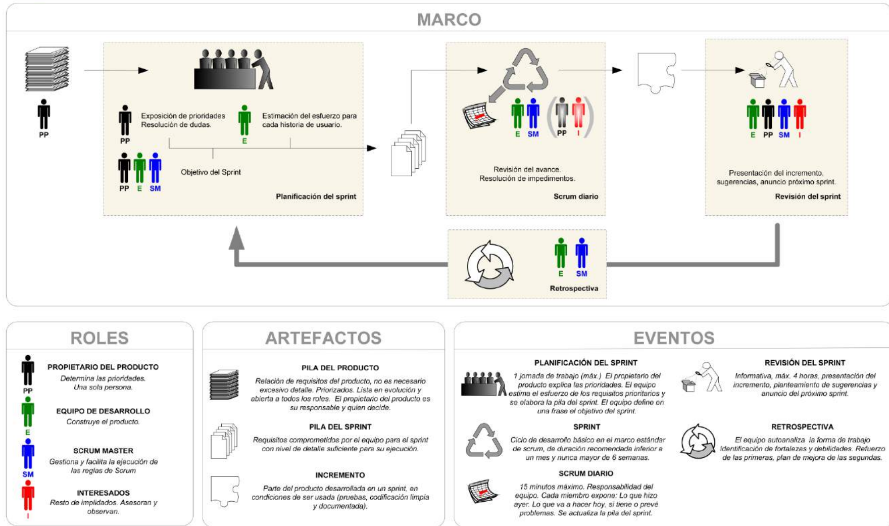
Ilustración 5: Marco scrum técnico
